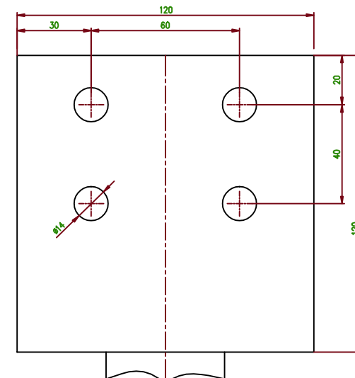
Připojovací kus FP M48
