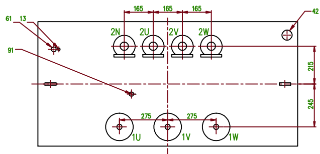
Pohled na víko
