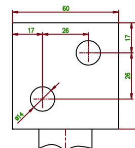
Připojovací kus EP M30
