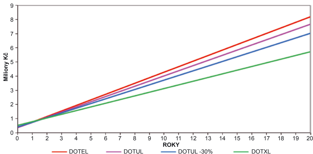
POROVNÁNÍ NÁKLADŮ U OLEJOVÝCH TRANSFORMÁTORŮ 1000 kVA S RŮZNÝMI ZTRÁTAMI
